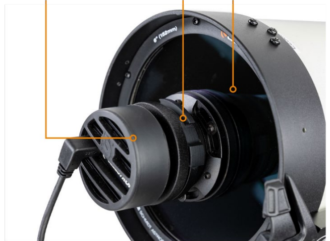
図14：フィルター引出しはカメラと補正板の間にあります。
