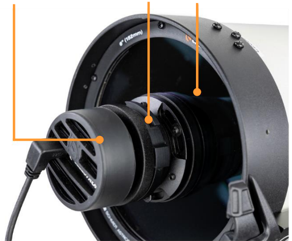
図14：フィルター引出しはカメラと補正板の間にあります。
